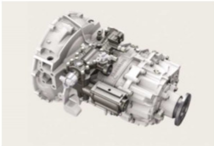
ZFecolite 5 / 6 단
